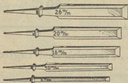
5 Stück starke Stechbeitel 1/2 lang, mit Fase, sortiert, für Wagner und Stellmacher. Breite: 6, 10, 16, 20, 26 mm. Preis per Satz RM 3.65
