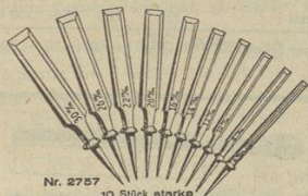
Nr. 2757 10 Stück starke Stechbeitel , 1/2 lang mit Fase, sortiert für Wagner und Stellmacher Breite 6 8 10 12 14 16 20 22 26 30 mm Preis per Satz RM. 7.25
