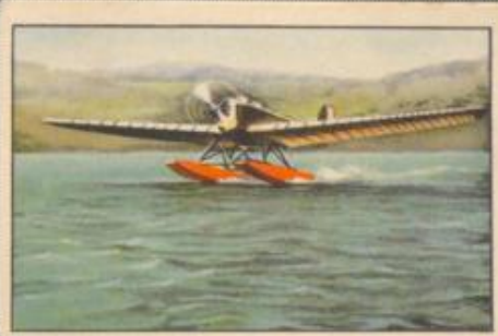
Nr. 4 Klemm WL 25 la 2 sitziges Sportflugzeug auf Schwimmern. 40-PS-Salmson AD 9 Motor, luftgekühlt.
