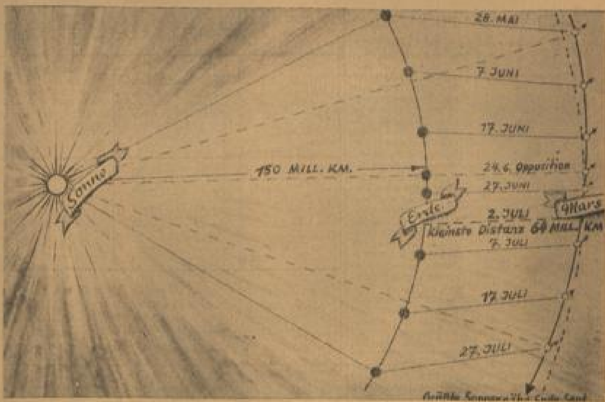
Sonne - Erde - Mars / Der „rote Stern“ hält keine Kreisbahn (s. die gepunktete Linie) ein. Er beschreibt (s. die durchgezogene Linie) eine Ellipse. Zeichnung: Flammig
