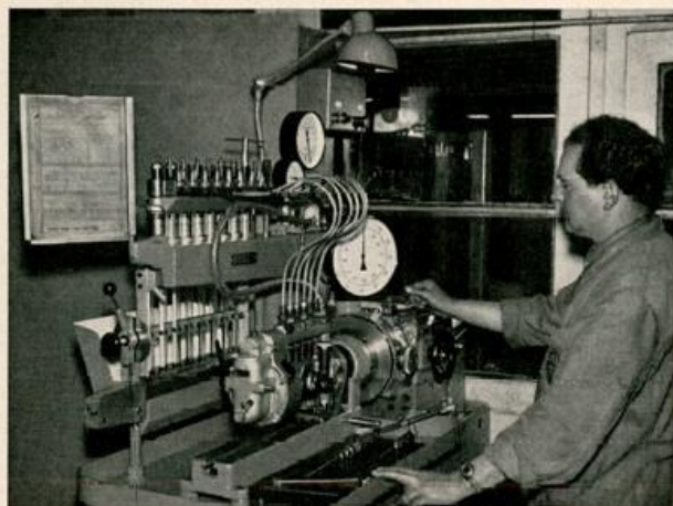
Am BOSCH-Diesel-Einspritzpumpenprüfstand
