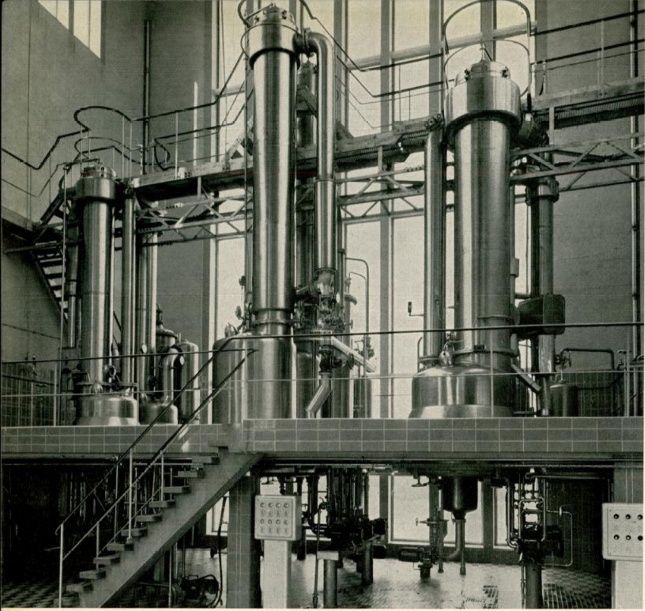
Drei 2-stufige Fallstrom-Verdampfer für Milch in Offenburg.
